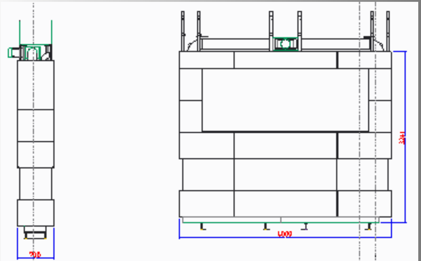
Abb. 3: Maßzeichnung
